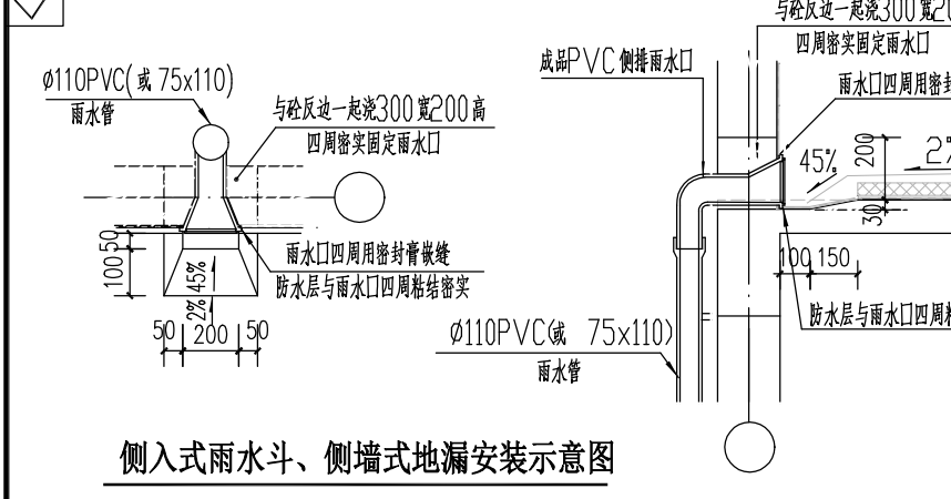
侧入式雨水斗、侧墙式地漏安装示意图
