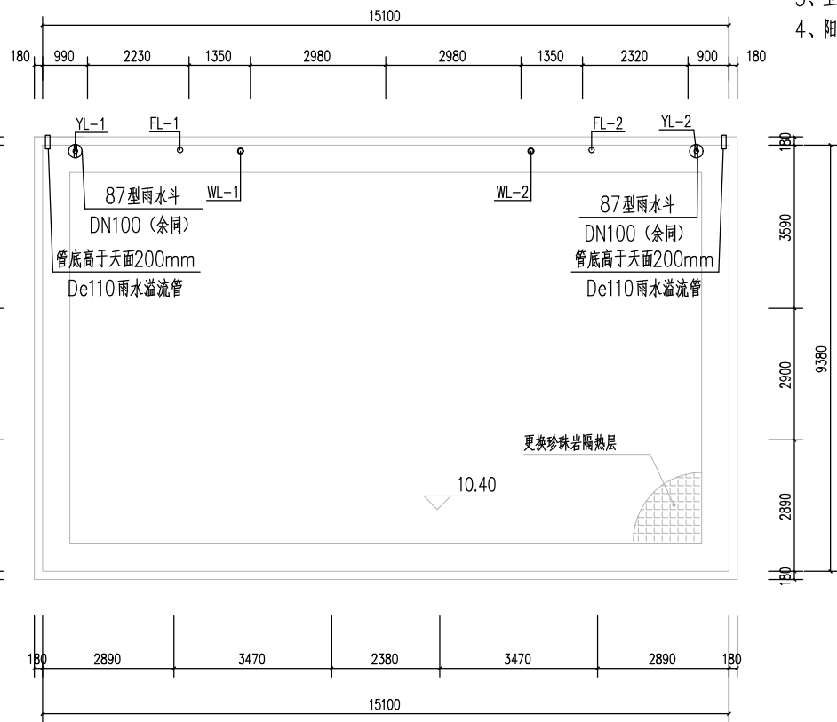
宿舍天面层给排水平面图 1:100
