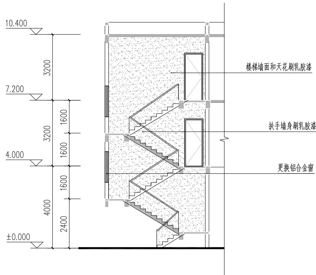
楼梯改造剖面图
