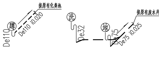
首层卫生间W1排水轴测图
