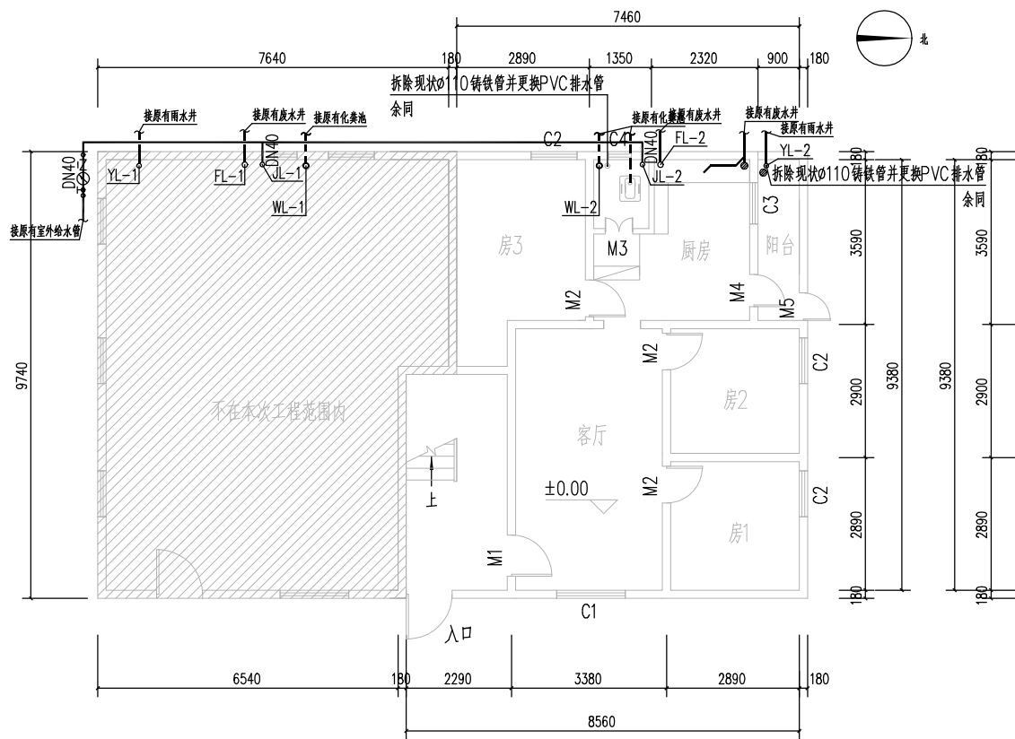
宿舍首层给排水平面图 1:100
