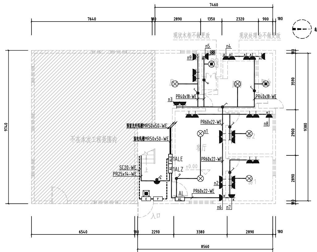
首层电气平面图 1:100
