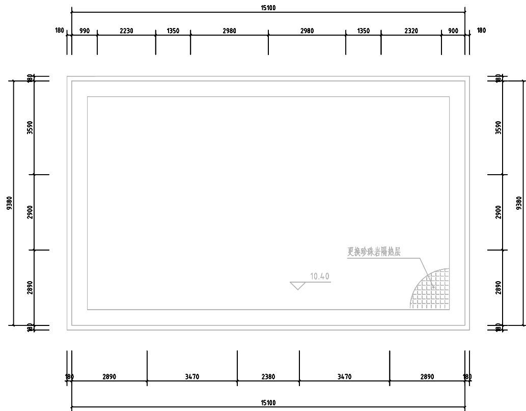
天面平面图 1:100
