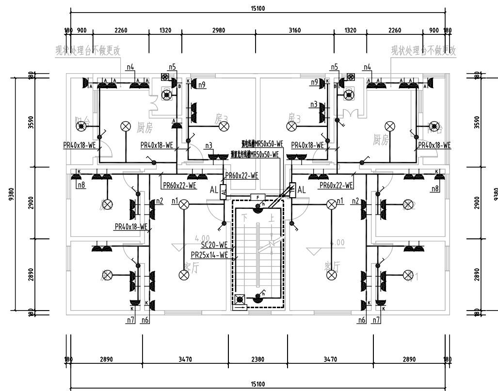
二层电气平面图 1:100
