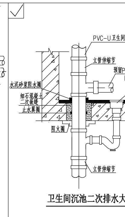
卫生间沉池二次排水大样
