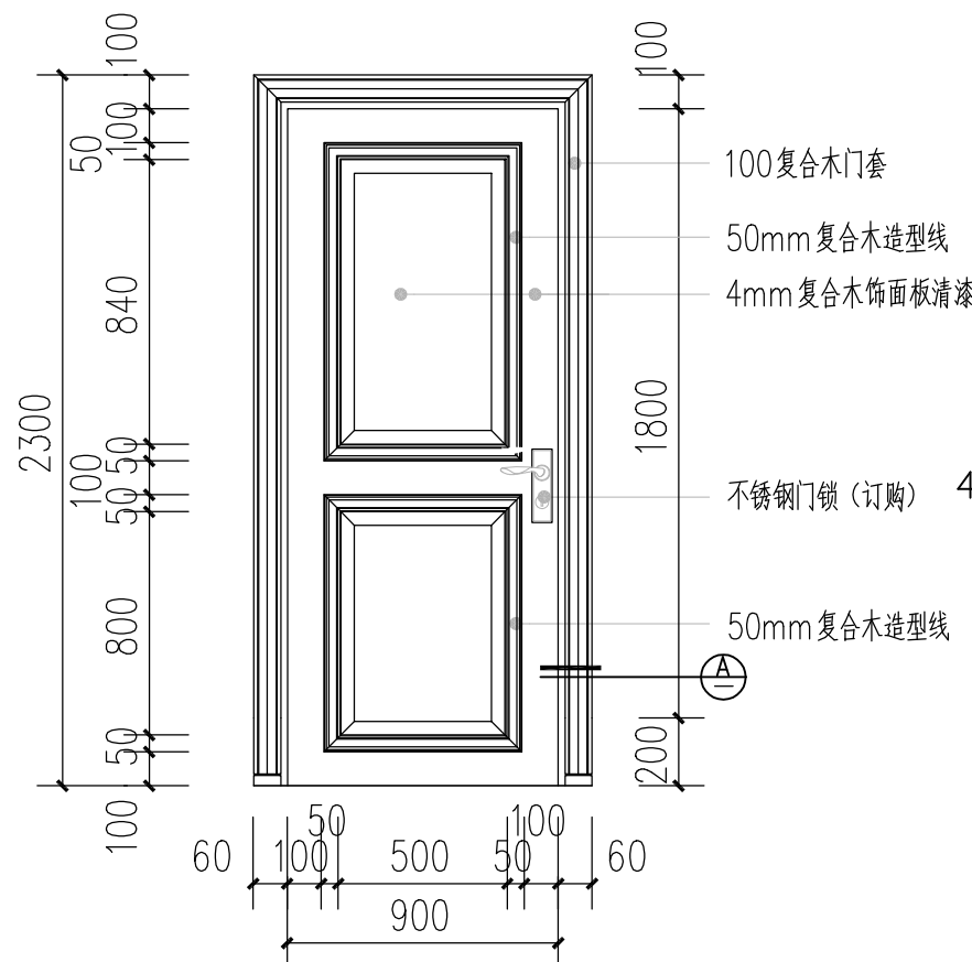
单扇平开木门大样图
