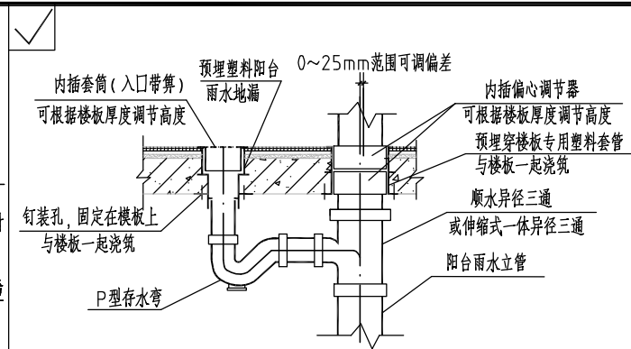
阳台雨水地漏、排水塑料管穿楼板安装
