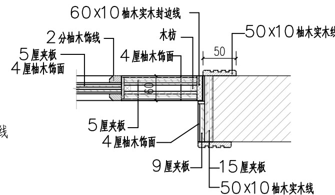
剖面图
