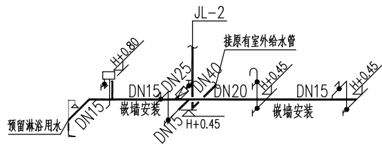
首层卫生间W1给水轴测图
