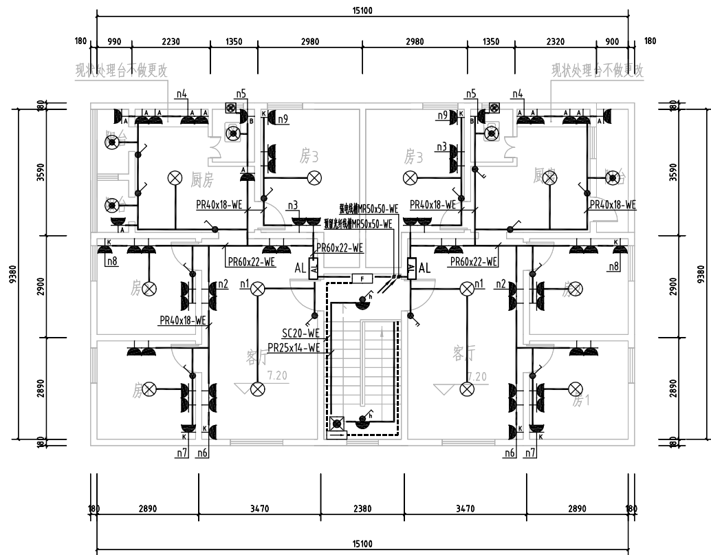
三层电气平面图 1:100
