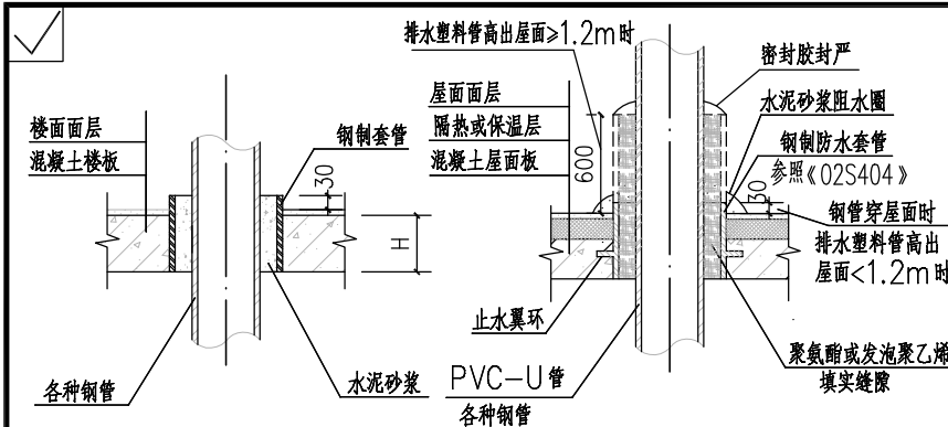
给水管穿管井、卫生间沉箱楼板 管道穿楼面、屋面大样图
