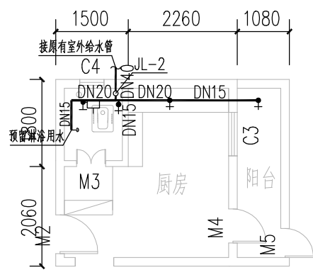
首层卫生间W1给水平面图 1:75
