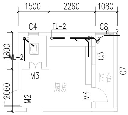
二层卫生间W2排水平面图 1:75
