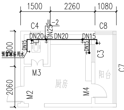
二层卫生间W2给水平面图 1:75
