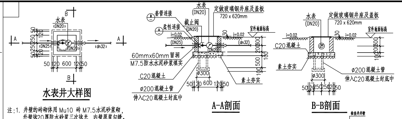
小型水表井安装
