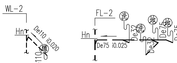
二层卫生间W2排水轴测图
