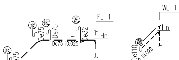
三层卫生间W3排水平面图 1:75
