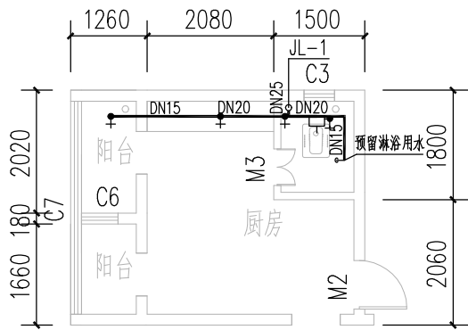
三层卫生间W3给水平面图 1:75
