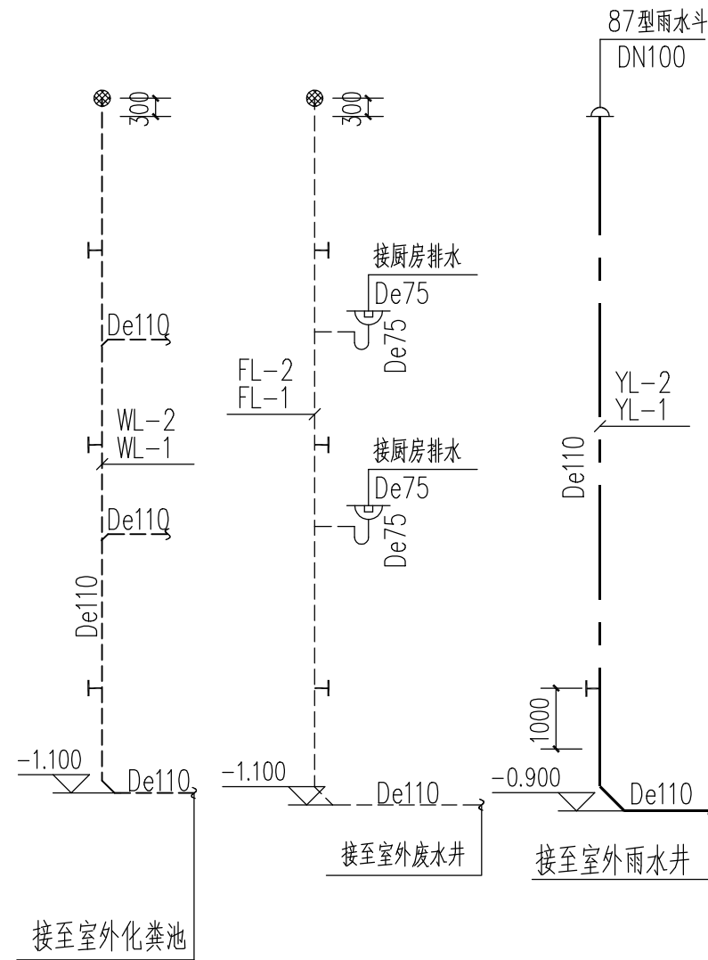
给排水系统示意图
