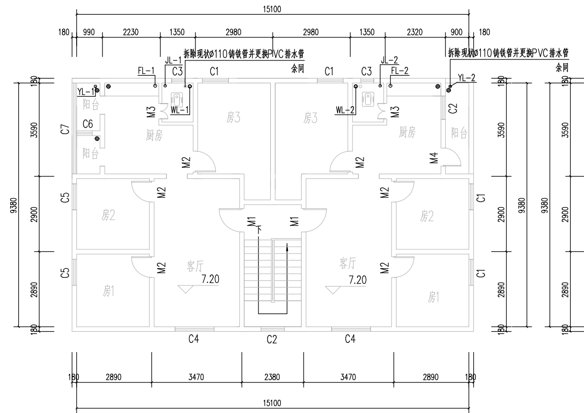
宿舍三层给排水平面图 1:100
