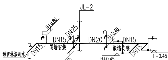
二层卫生间W2给水轴测图
