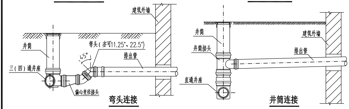
污水出户管道与塑料检查井的井座、井筒连接示意图
