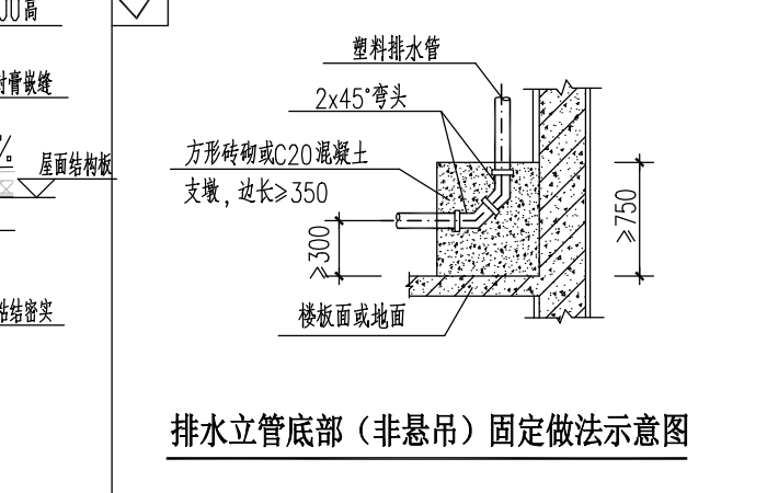
排水立管底部(非悬吊)固定做法示意图
