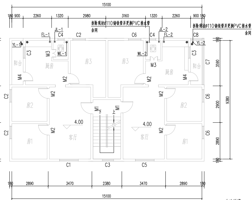
宿舍二层给排水平面图 1:100
