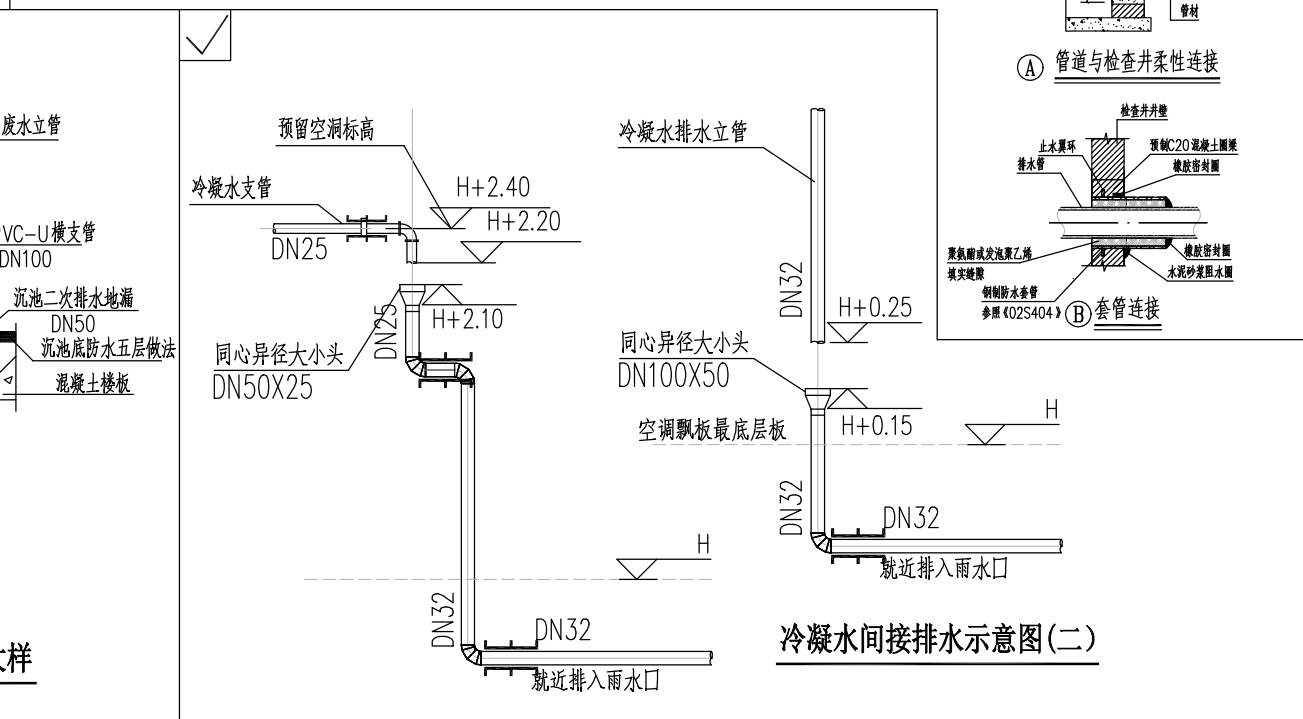
冷凝水间接排水示意图(一)
