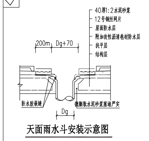
屋面雨水斗安装示意图
