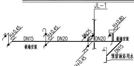
三层卫生间W3给水平面图 1:75
