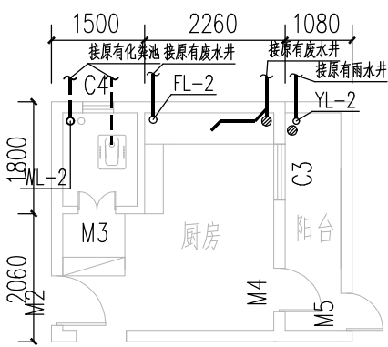
首层卫生间W1排水平面图 1:75
